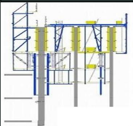
高层爬升模板施工
