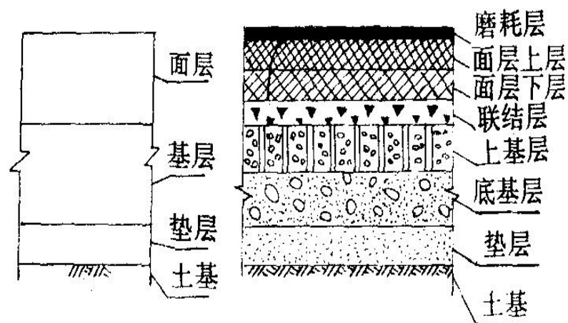
路面结构层
