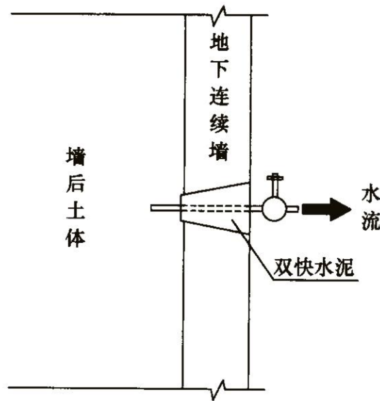
图1K420151-1 基坑围护墙体堵漏方法
