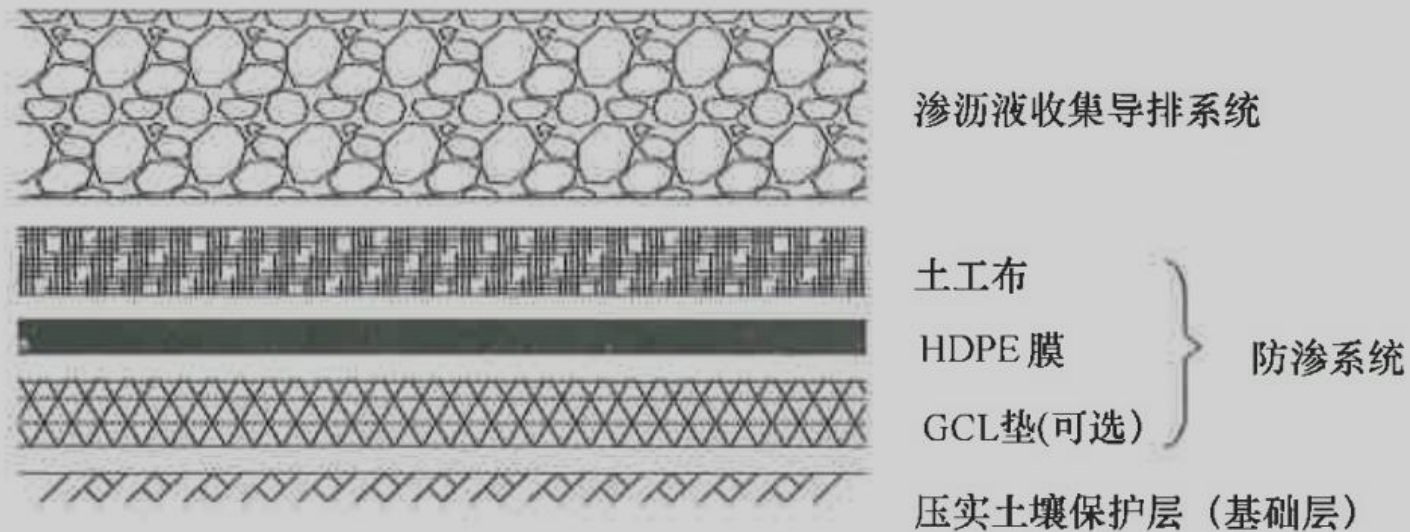
渗沥液防渗系统、手机导排系统断面示意图
